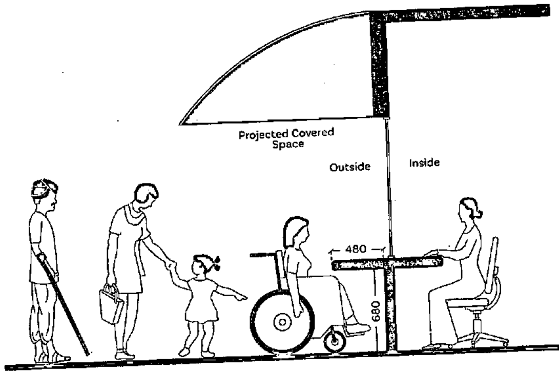
Fig a: Section
