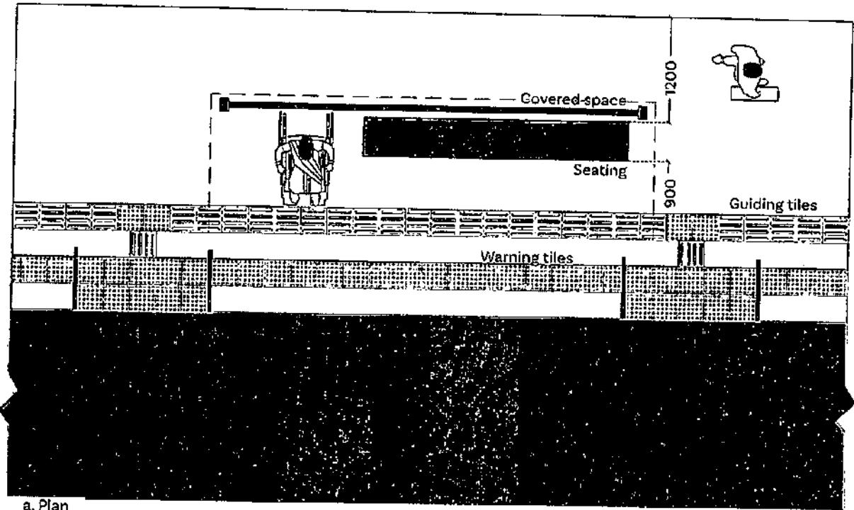
a. Plan
